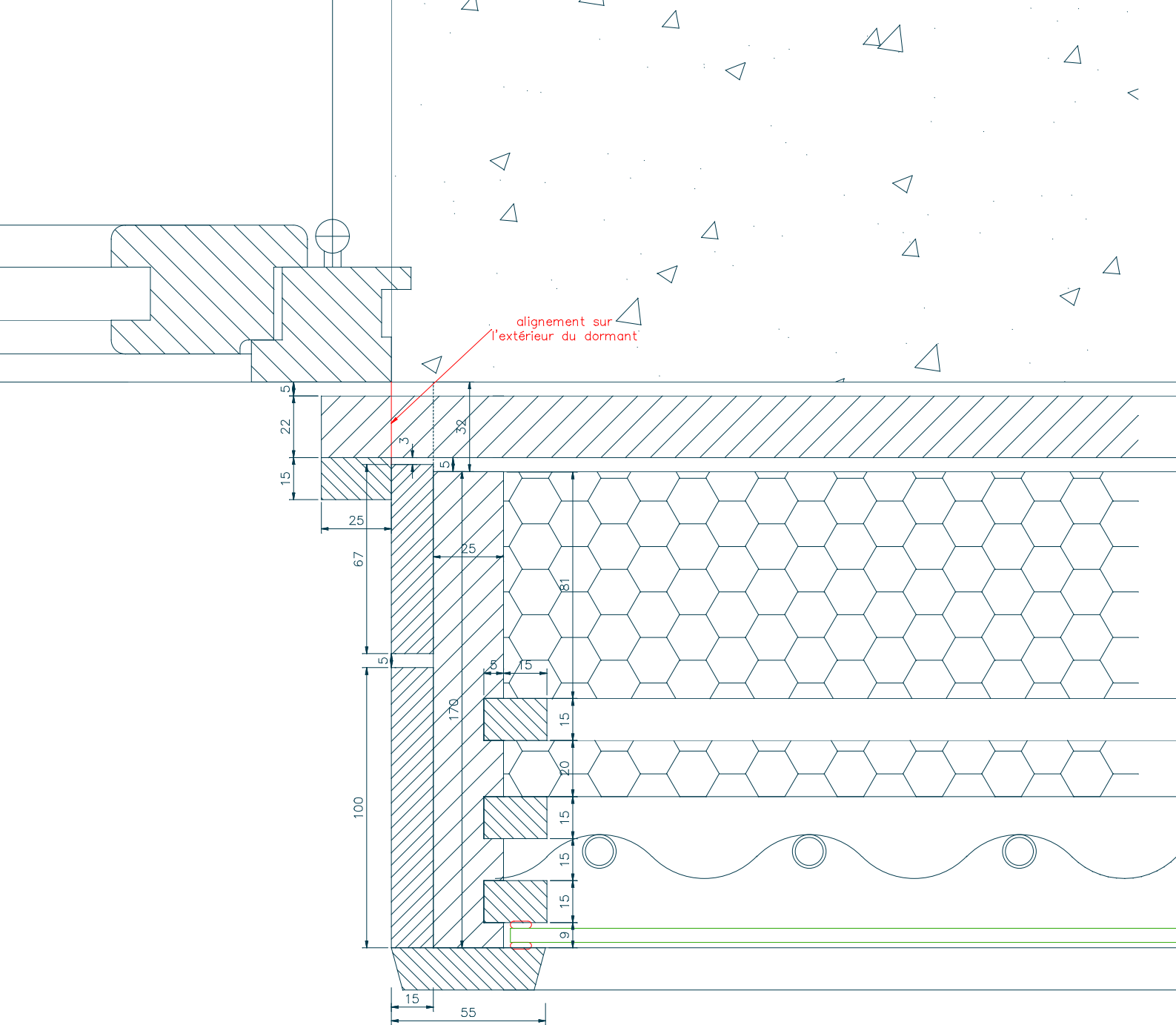
détails du raidisseur-butée vertical du volet en bois dur 30x50 long 1932mm (coté intérieur du coffre)
